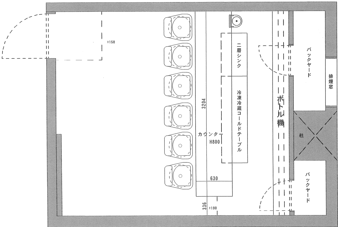
店舗平面図
